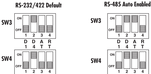
Figure 3-6. RS-485 Enable modes.
