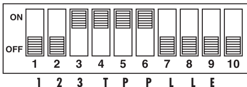
Figure 3-2. RS-422.
